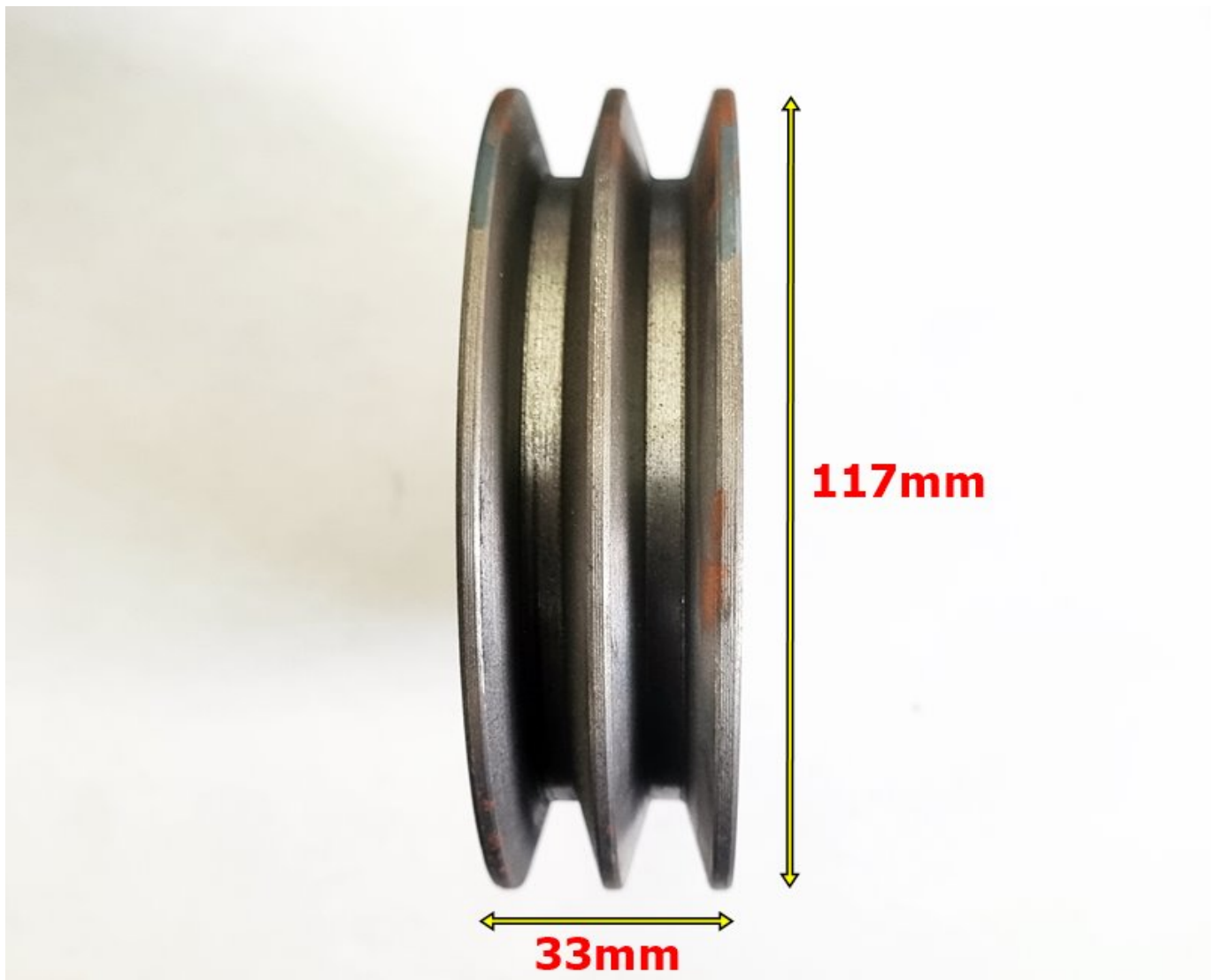
SCHEMAT ROZDRABNIACZA SPALINOWEGO XARAM Garden seria TPS 700, TPS750, TPS1300, TPS1500 - koło pasowe duże poz. 42
